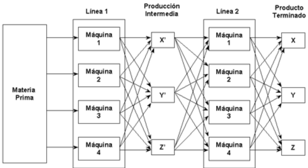
Figura 2.1 El Proceso de Producción de SIMPRO
